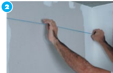
2 Marcado de la posición de los perfiles perimetrales Con el auxilio de un hilo entizado (chocla), marcar la posición exacta donde será fijado el perfil perimetral L.
