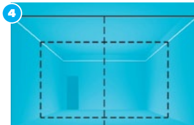
4 Establecer ejes de replanteo Definir con una tanza los ejes de replanteo tomando como unión el centro del local. Luego, adaptar la modulación de la estructura, ubicando las placas recortadas en el perímetro y preferentemente en forma simétrica.
